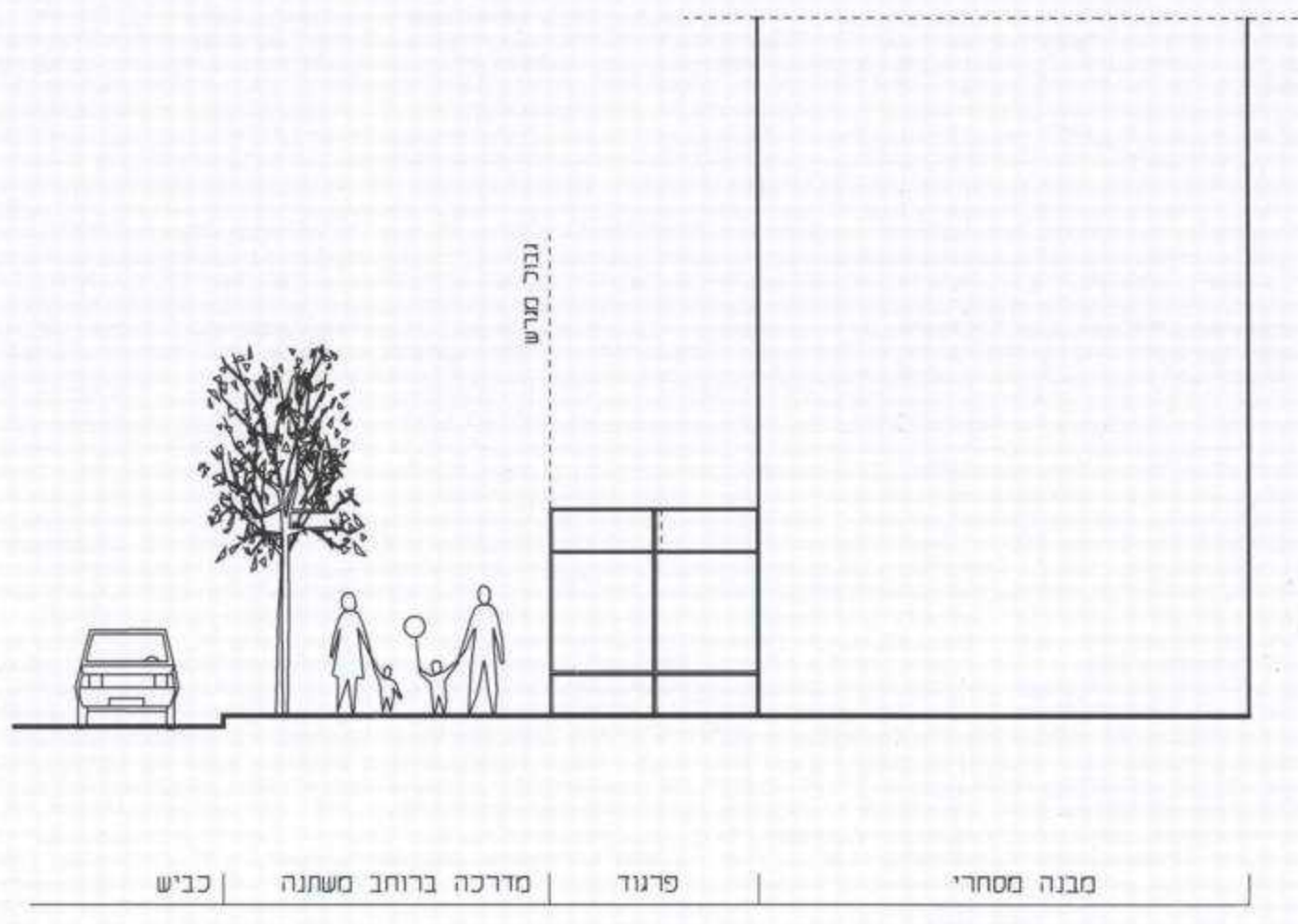
חלופה ג' | בנית פרגוד בתחום המגרש
