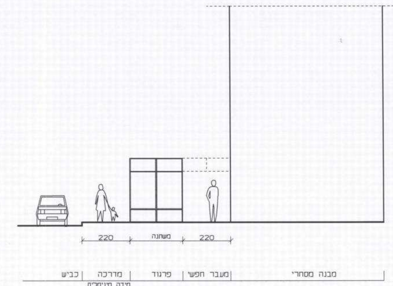
חלופה א' | בנית פרגוד בתחום המדרכה
